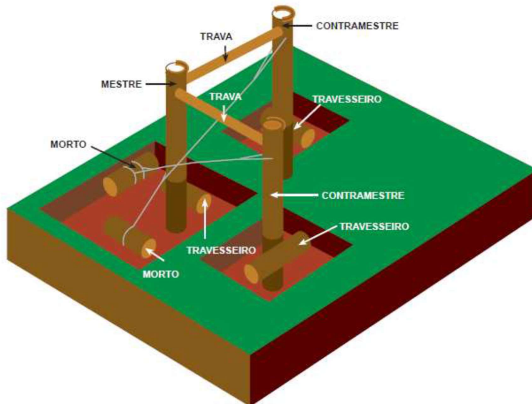
Figura 3: Desenho do canto duplo em ângulo.
