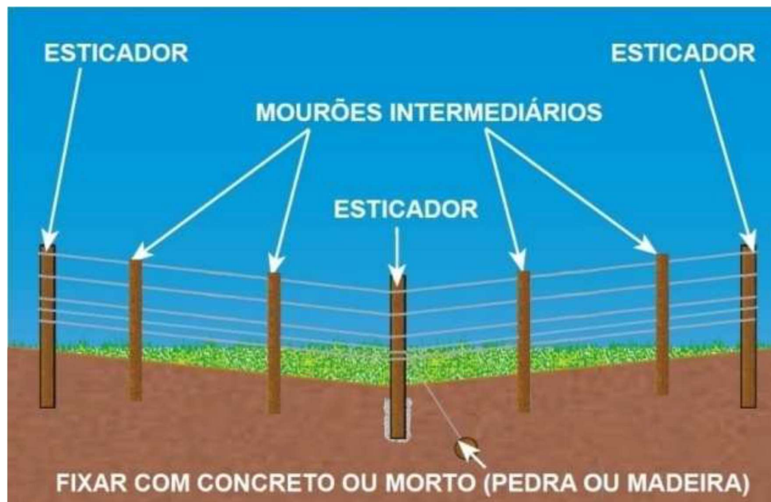
Figura 4: Croquis de mourão para área com depressão acentuada.
