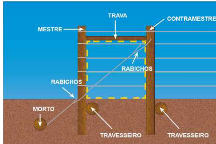
Figura 2: Croquis de canto duplo.
