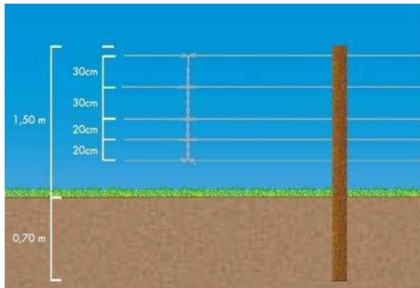
Figura 1: Croquis das características das cercas.
