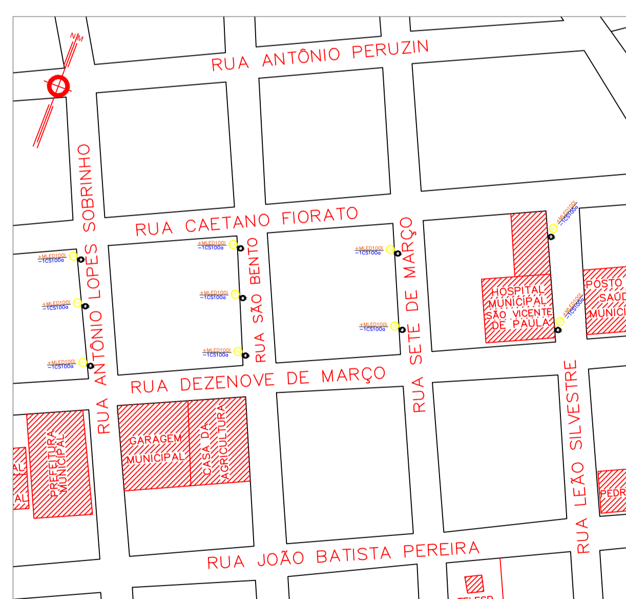
TRECHO 2 ESC. 1:2000
